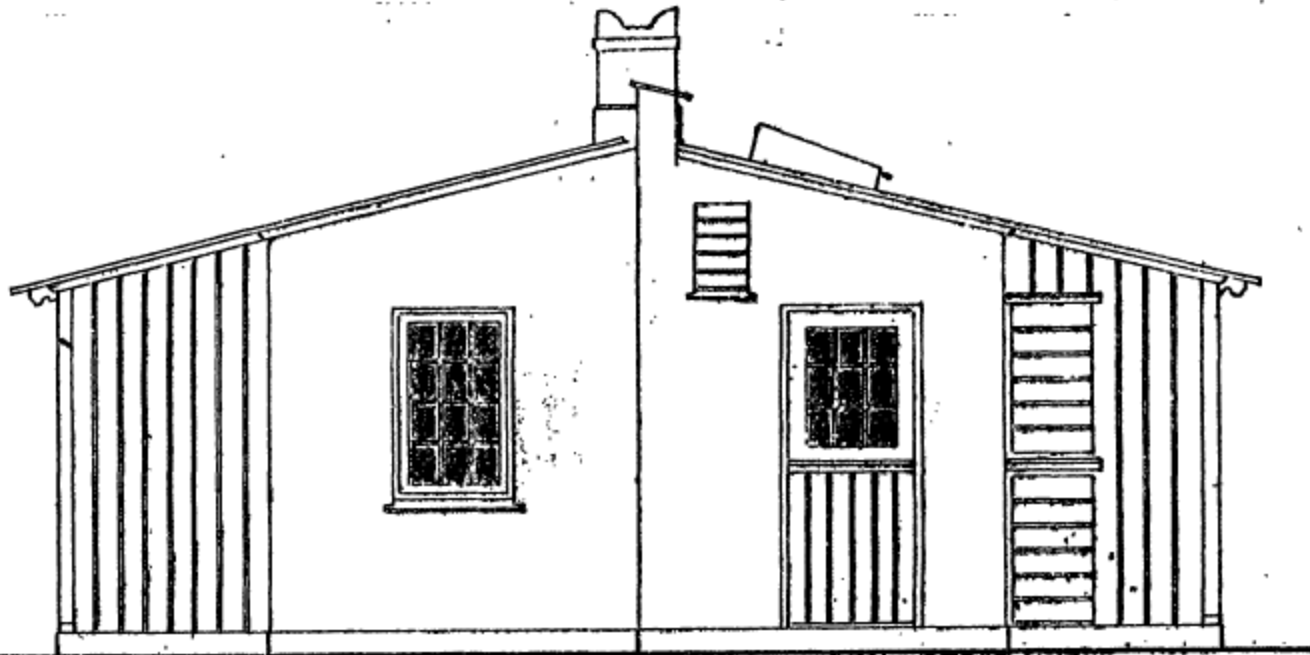
Snit C-D.
