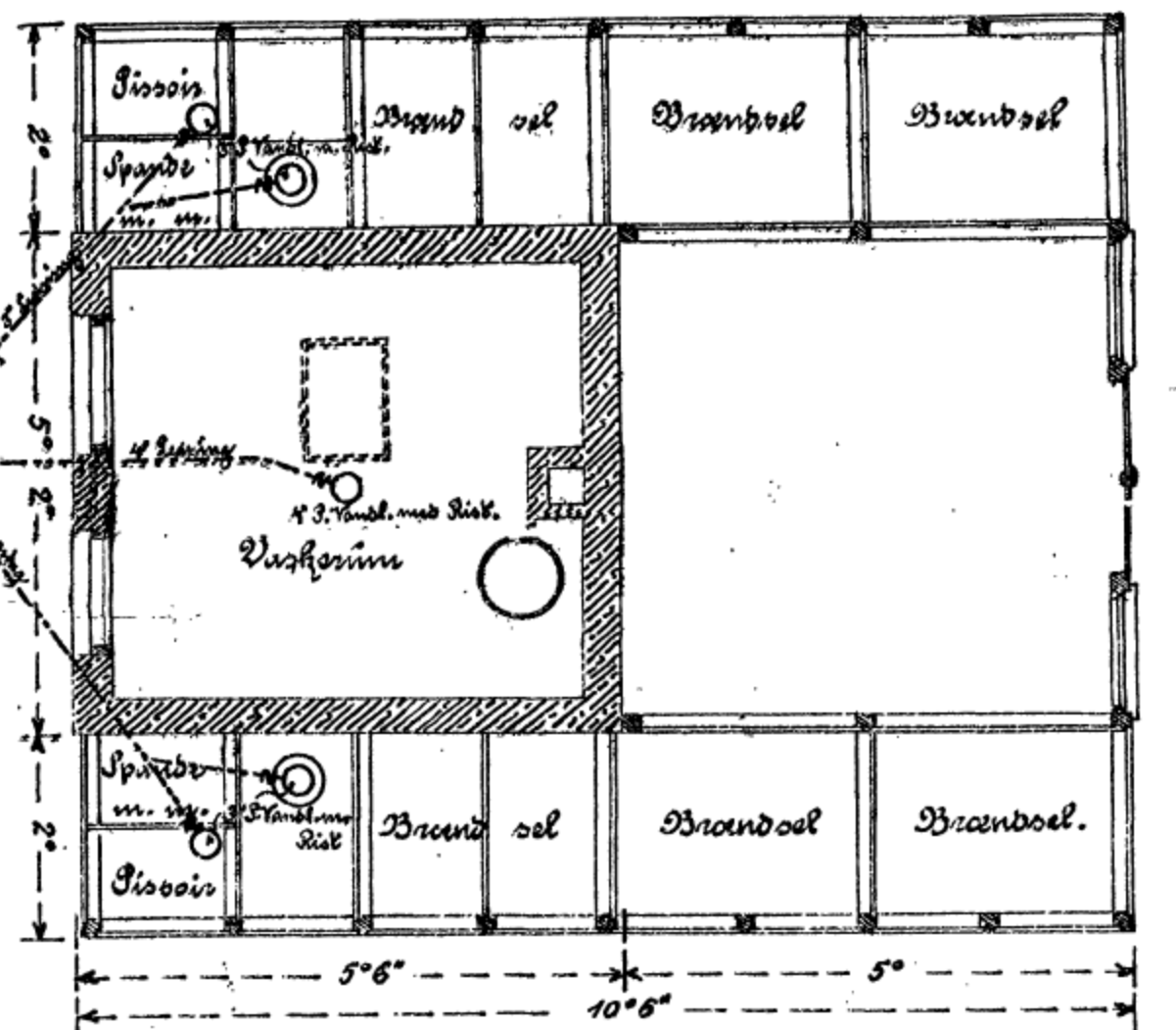
Plan of Type VI. 1 Skk.
