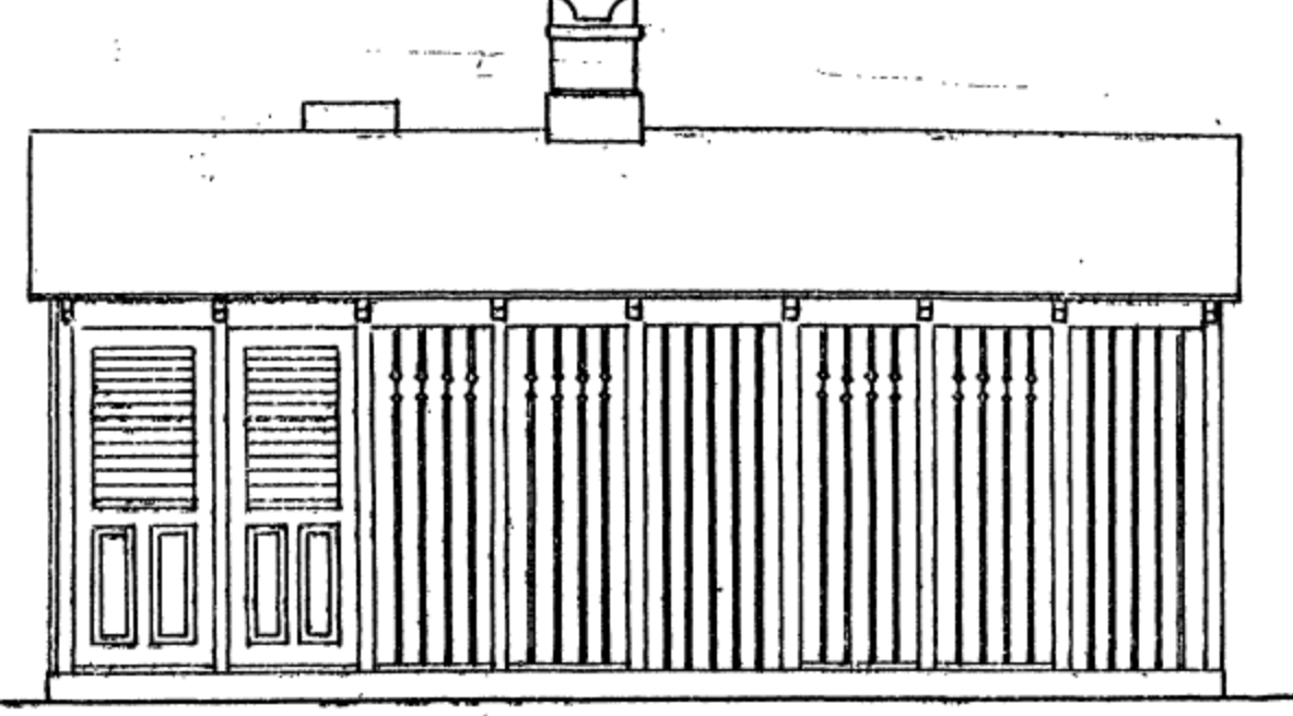
Facade.
