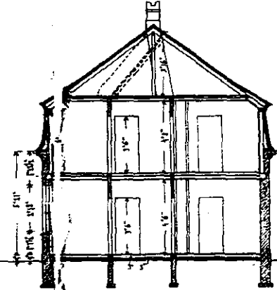
Længderisning
